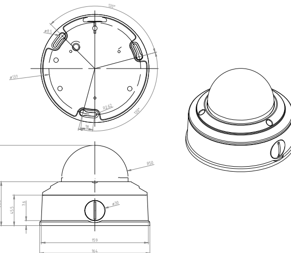
Камера наблюдения цифровая купольная
