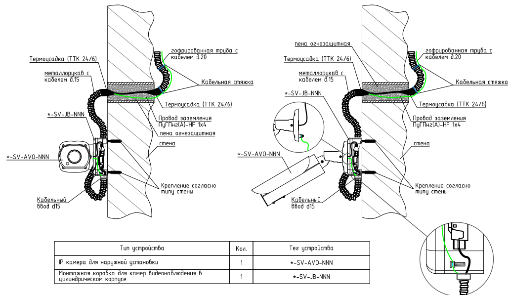
Узел крепления наружной видеокамеры
