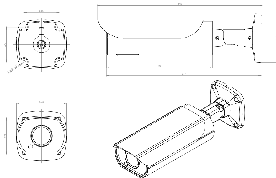
Камера наблюдения цифровая цилиндрическая
