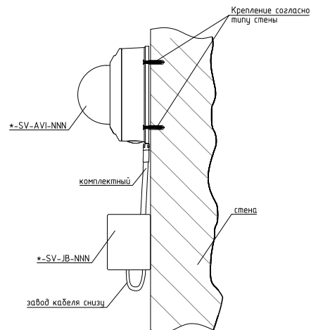
Узел крепления внутренней видеокамеры к стене
