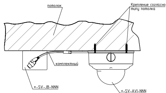
Узел крепления внутренней видеокамеры к потолку
